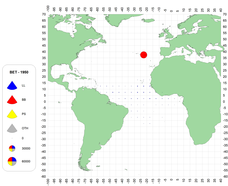
a. BET(1950-1959)
