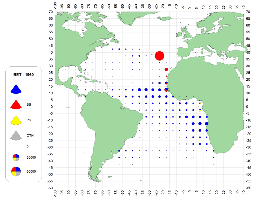
b. BET(1960-1969)
