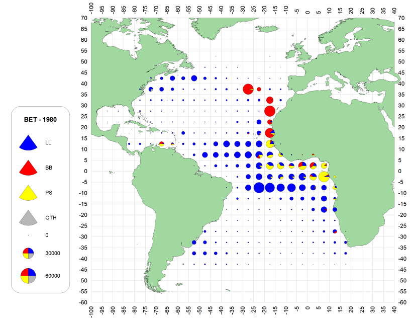
d. BET(1980-1989)
