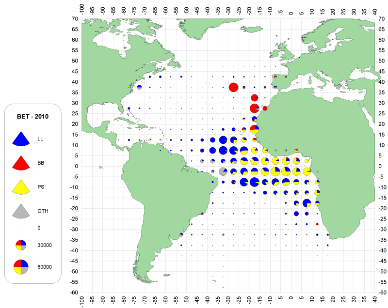
g. BET (2010-2019)
