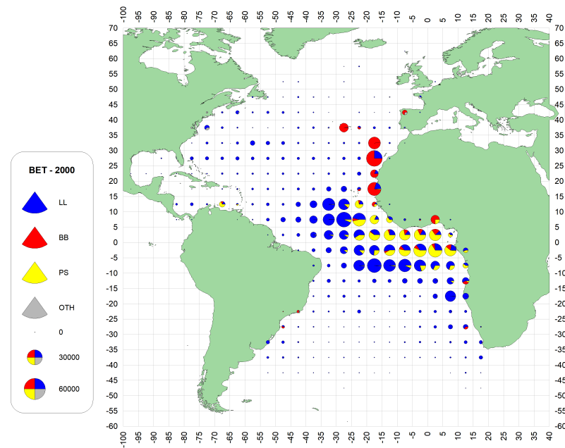
f. BET (2000-2009)
