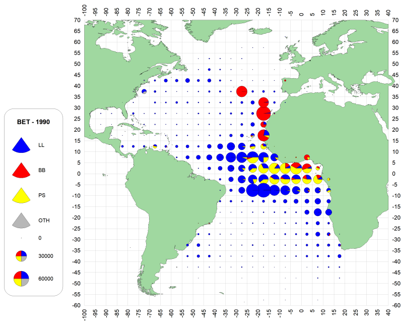
e. BET (1990-1999)
