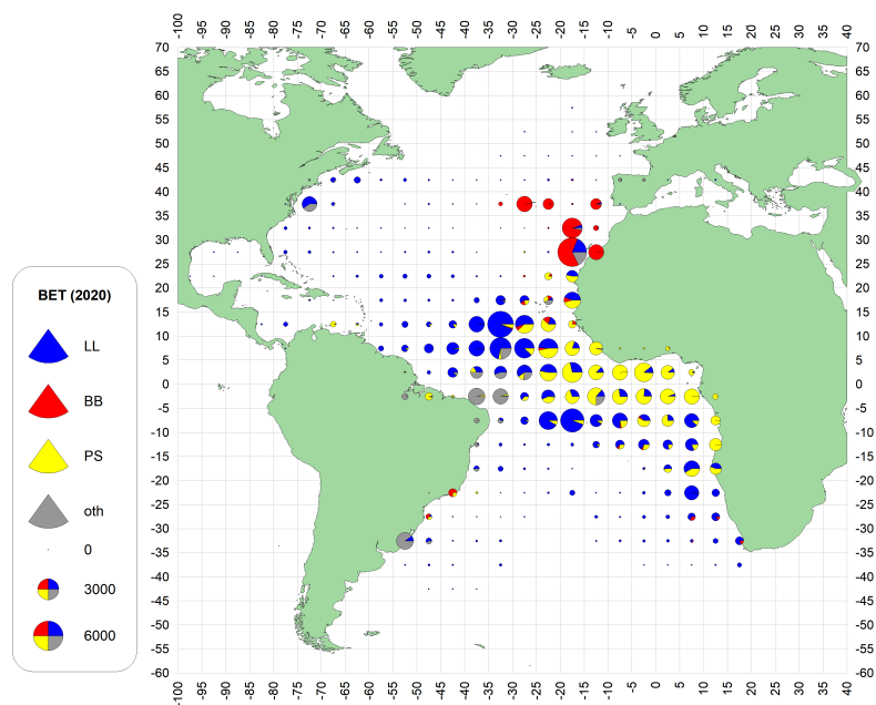
h. BET (2020-2021)
