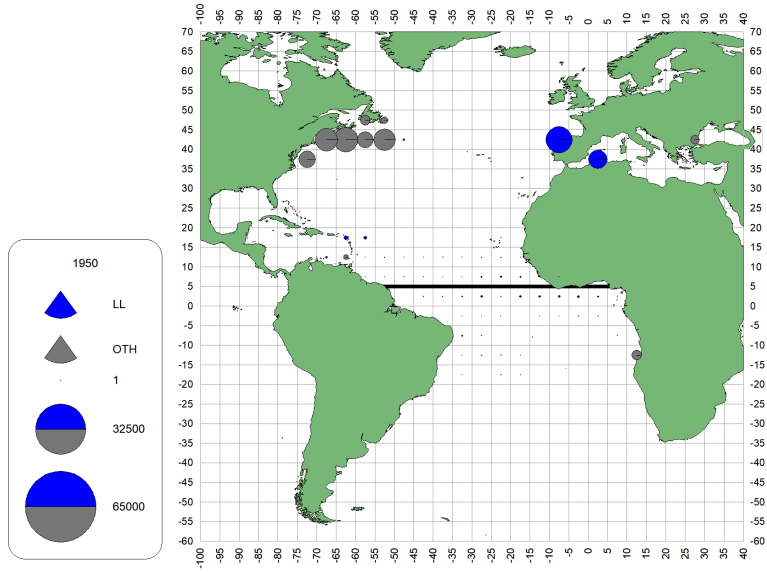
a. SWO(1950-59)
