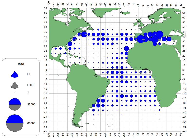
g. SWO (2010-17)
