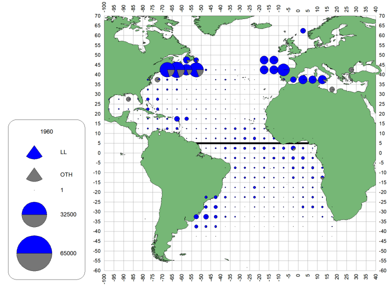
b. SWO (1960-69)
