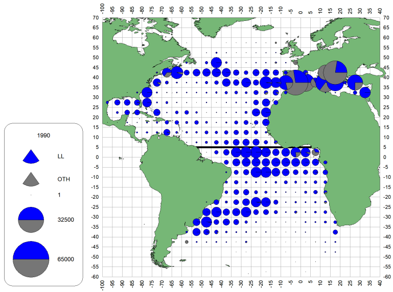
e. SWO (1990-99)
