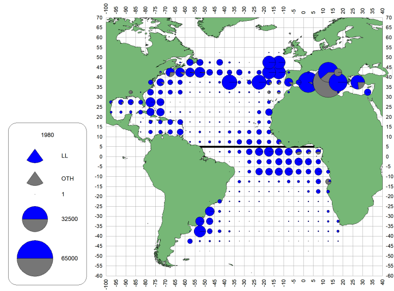
d. SWO (1980-89)
