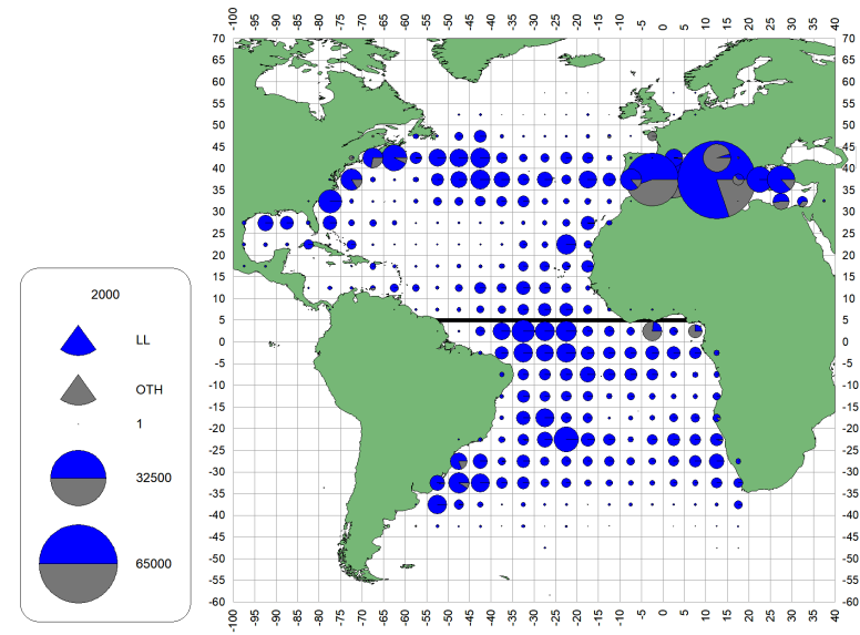
f. SWO (2000-09)
