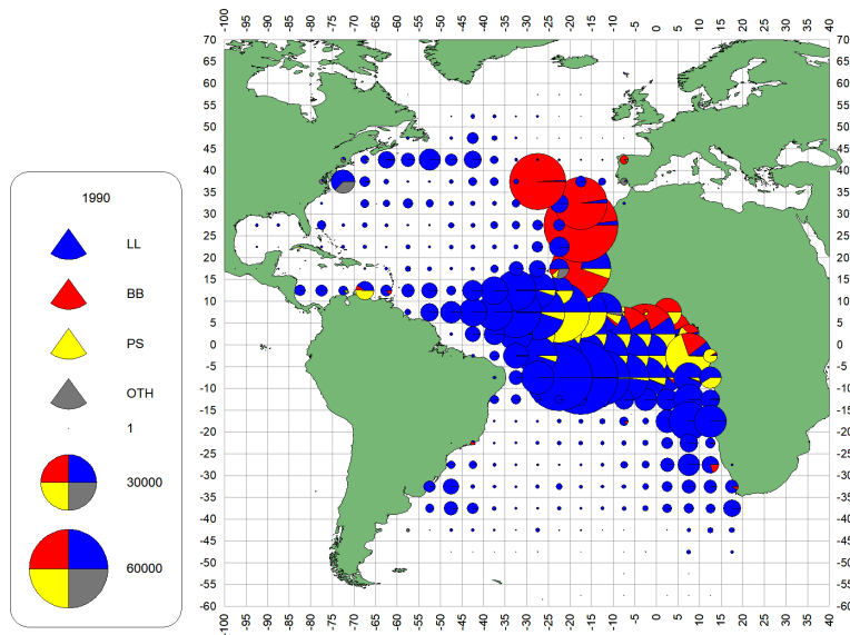
e. BET (1990-99)
