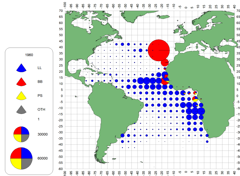
b. BET(1960-69)
