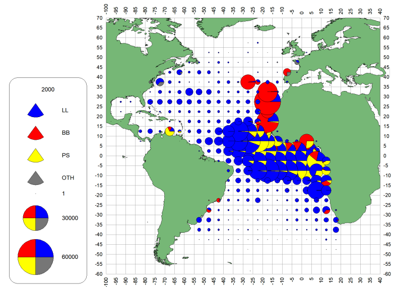
f. BET (2000-09)
