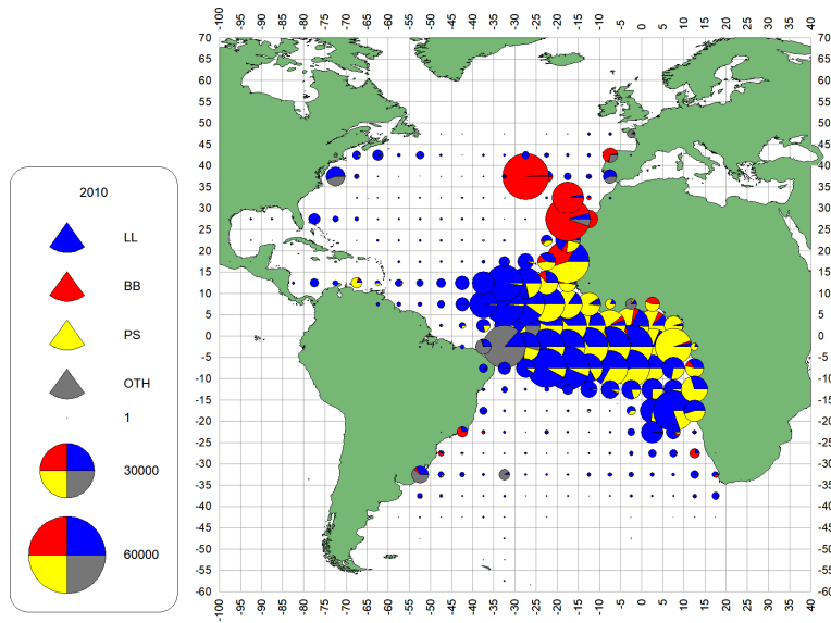
g. BET (2010-17)
