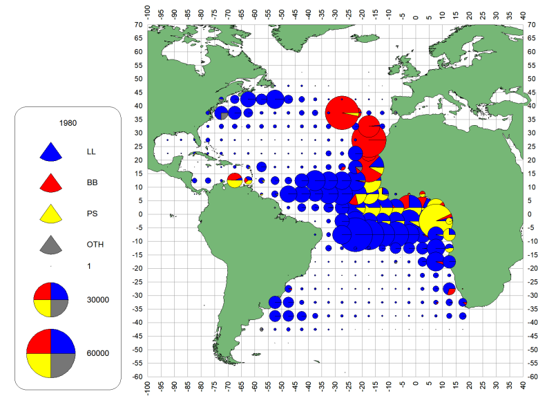
d. BET(1980-89)
