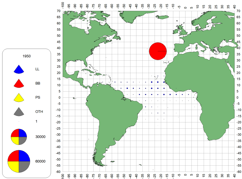
a. BET(1950-59)
