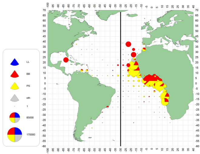
b. SKJ(1970-79)
