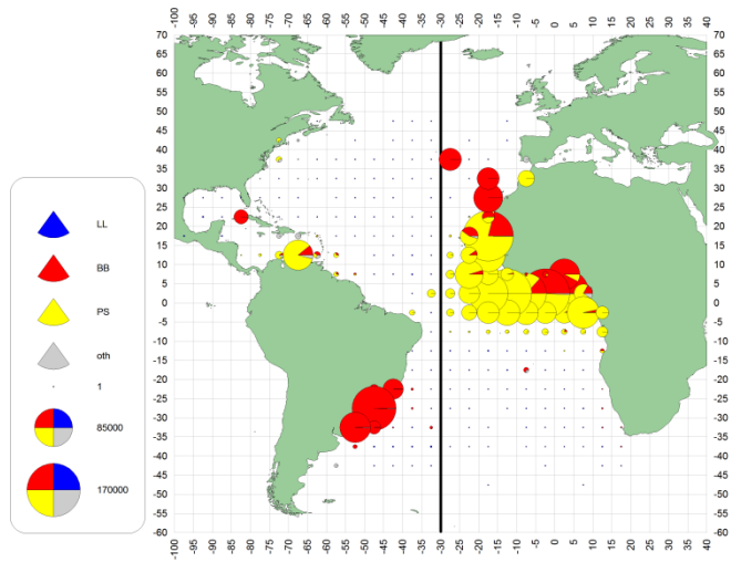
d. SKJ(1990-99)
