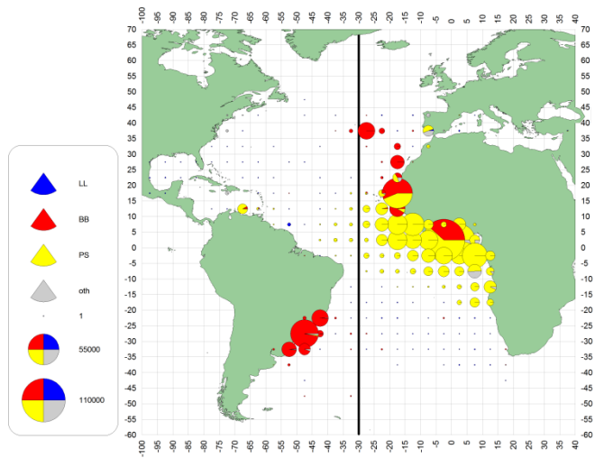
f. SKJ(2010-12)
