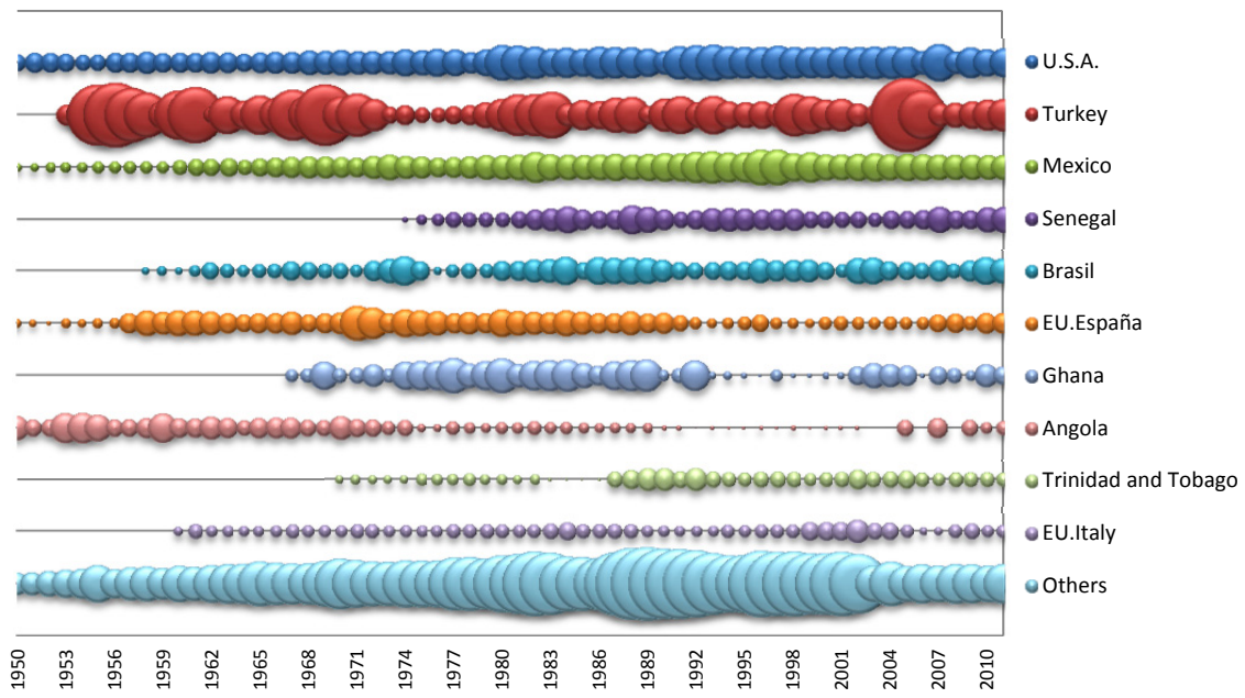
Figure 43 Relative other tunas catch distribution by major Fleets. Ranking of catches based on the average amount of the five previous years. Figure 43 Distribution relative de la prise de autres thonidés par flottille principale. Classification des captures sur la base de la moyenne des cinq dernières années. Figura 43 Distribución relativa de la captura de otros túnidos por flotas principales. Clasificación de capturas en base a la media de los cinco últimos años.
