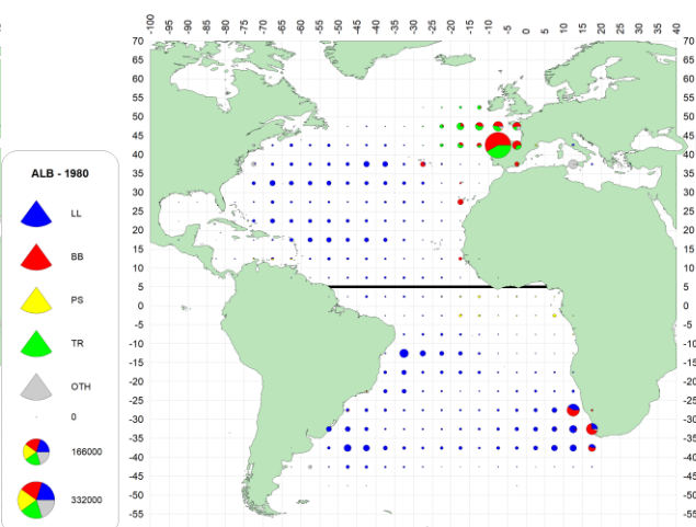
b. ALB (1980-89)
