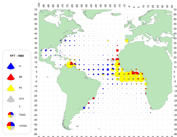
g. YFT (1980-89)
