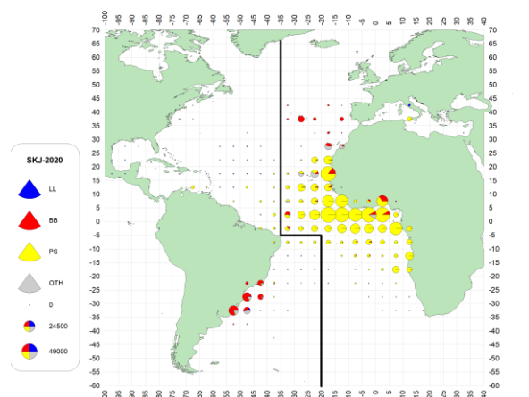
f. SKJ (2020-22)
