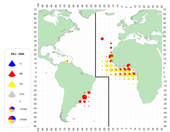
d. SKJ (2000-09)
