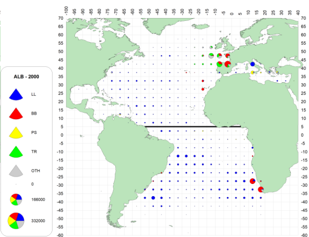
d. ALB (2000-09)
