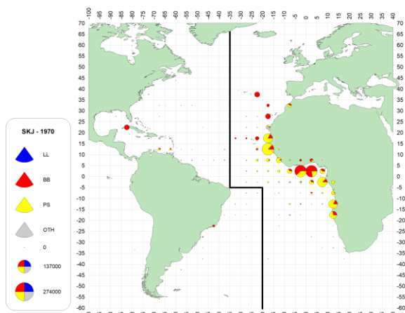
a. SKJ (1970-79)
