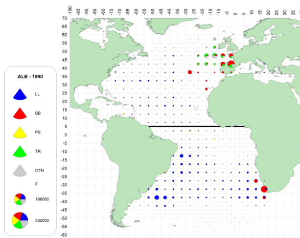
c. ALB (1990-99)
