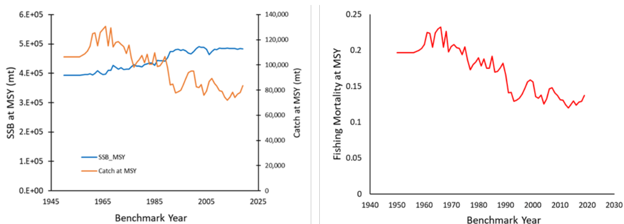
BET-Figura 9. Dinámica SSB/SSB_{RMS} y capturas en RMS (panel de la izquierda) y F/F_{RMS} (panel de la derecha) por año de referencia, demostrando los efectos de los cambios en la selectividad del patudo utilizando el caso de referencia Stock Synthesis de 2021.
