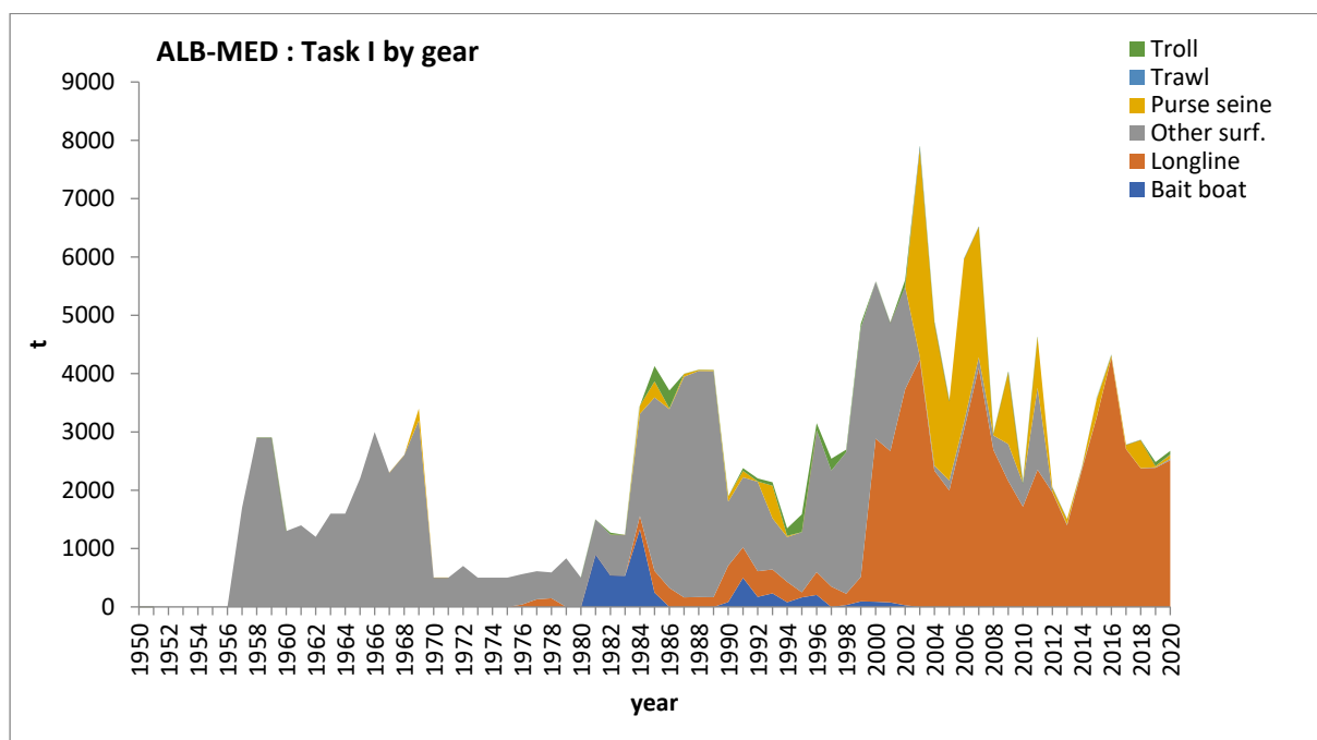
ALB-figure 2. Prises totales de germon déclarées à l'ICCAT (tâche 1) par engin pour le stock de la Méditerranée.
