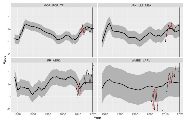
Figure 21.24.2. Indices actualisés (valeurs postérieures à 2019, ligne noire) comparés aux intervalles de prédiction de 80% de la VPA de 2017 projetés en avant avec les captures observées et le recrutement moyen sur 6 ans. Les points rouges sont les indices utilisés dans l'évaluation et les points noirs sont les valeurs actualisées ou révisées des indices. Les lignes noires épaisses représentent la tendance centrale de la composante de la population correspondant à l'indice. Pour interpréter les implications des points situés en dehors des intervalles de 80%, 20% des observations pourraient se situer en dehors de l'intervalle de façon aléatoire. Il est à noter que la méthodologie utilisée pour produire l'indice larvaire de la Méditerranée occidentale a été considérablement révisée depuis l'évaluation du stock de 2017, ce qui a produit des fluctuations notablement différentes entre les indices originaux et les indices actualisés.
