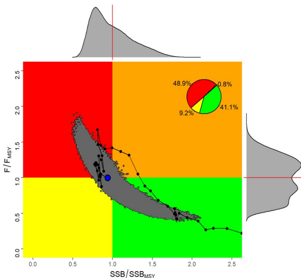
BET-figure 8. Stock Synthèse : Diagramme de Kobe de la SSB/SSB_{PME} et de la F/F_{PME} pour l'état du stock de thon obèse de l'Atlantique en 2019 sur la base de l'approximation normale multivariée logarithmique pour les 27 scénarios du modèle de la grille d'incertitude de Stock Synthesis avec un graphique circulaire inséré montrant la probabilité de se trouver dans le quadrant rouge (48,9%), le quadrant vert (41,1%), le quadrant orange (0,8%) et le quadrant jaune (9,2%). Le cercle bleu représente la médiane et les histogrammes marginaux représentent la distribution de SSB/SSB_{PME} ou de F/F_{PME} .
