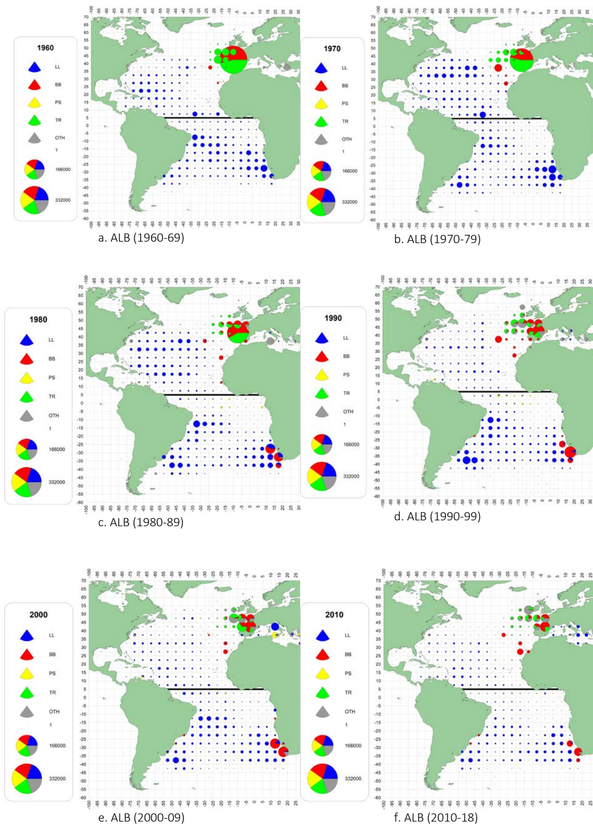
ALB-figure 1. Distribution géographique des captures cumulées de germon par engins principaux et décennie (1960-2018). Avant la décennie des années 90, les prises à la canne et à la ligne traînée ont été assignées à un seul carré de 5x5° dans le golfe de Gascogne. Les diagrammes sont échelonnés à la prise maximale observée entre 1960 et 2018 (la dernière décennie ne couvre que 9 ans).
