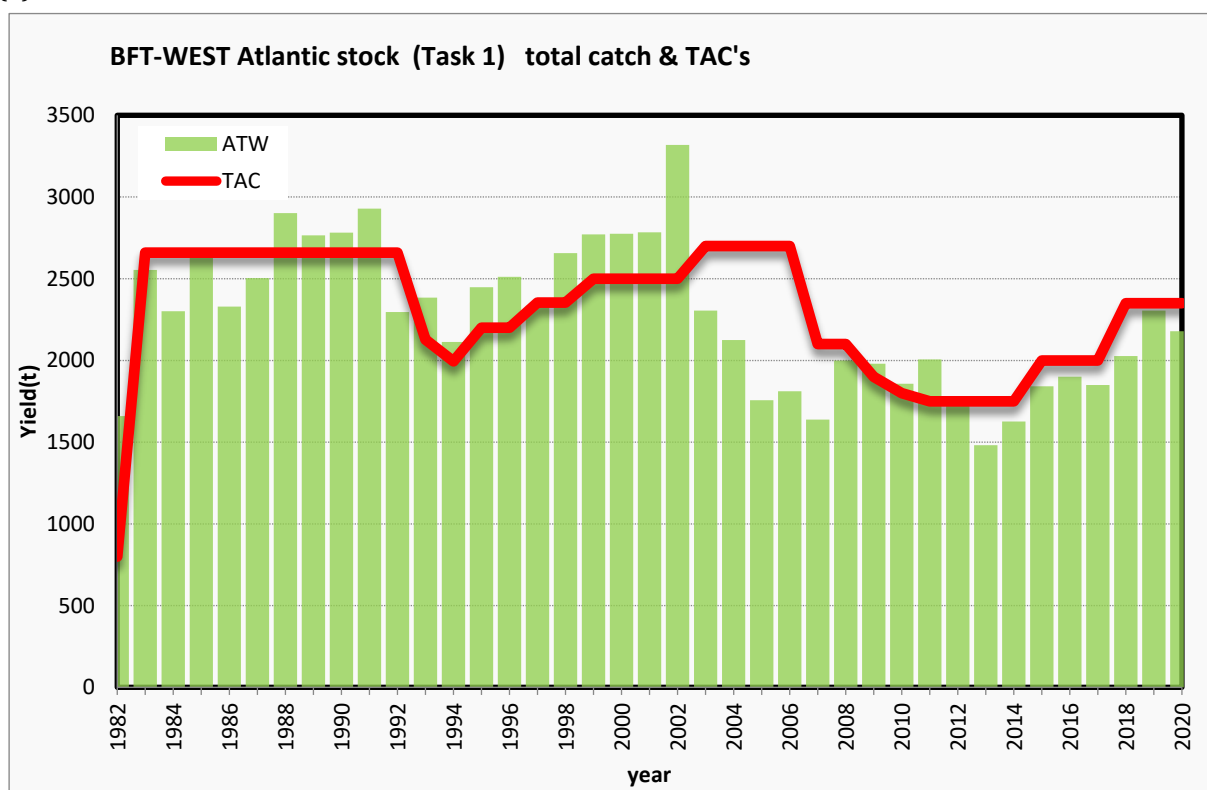
BFTW-figure 1. Prises historiques de thon rouge de l'Ouest : (a) par type d'engin et (b) TAC convenus par la Commission (présentés à des fins de comparaison).
