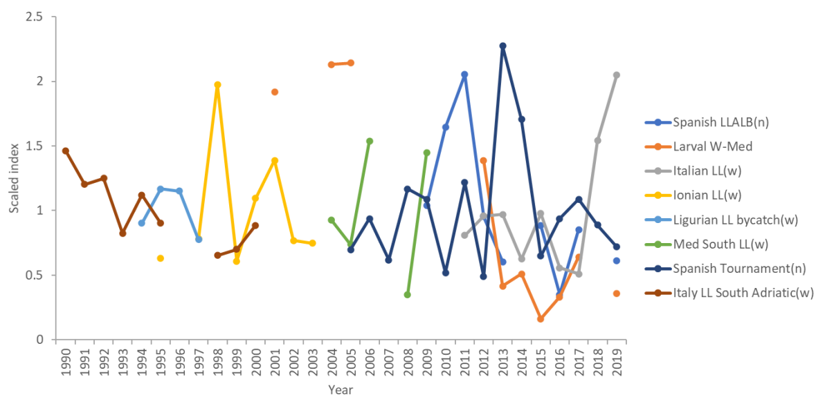
ALB-figure 3. Germon de la Méditerranée. Indices d'abondance utilisés dans l'évaluation de 2021 du stock de germon de la Méditerranée (Anon. sous presse). n et w désignent les indices d'abondance en nombre et en poids, respectivement.
