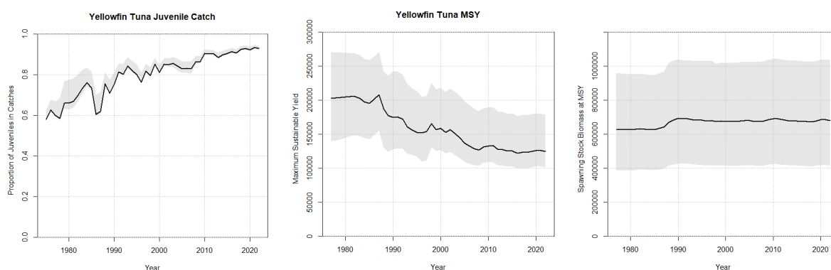
Figura 5. Proporción estimada (en número) de juveniles (edades 0, 1 y 2) en las capturas de rabil a lo largo del tiempo (gráfico de la izquierda) comparada con las estimaciones dinámicas en el tiempo del RMS (gráfico central) y biomasa dinámica del stock reproductor en RMS (gráfico de la derecha). El área sombreada representa los intervalos de confianza del 80 % del modelo de evaluación de matriz de incertidumbre.
