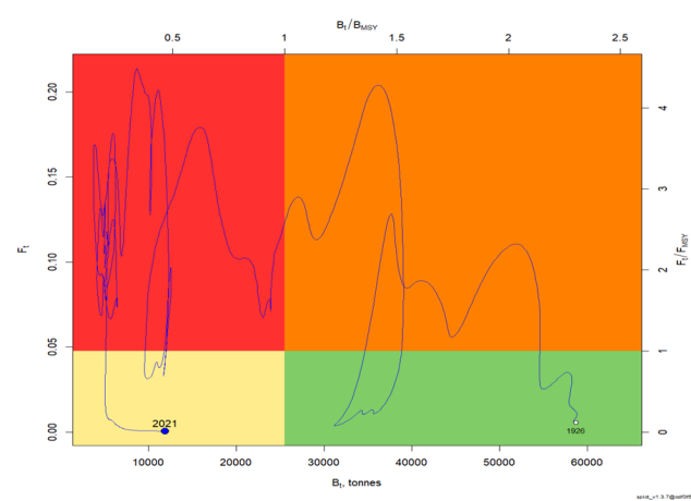
Figura 1. Diagrama de Kobe para el estado del stock de marrajo sardinero del Atlántico nororiental en 2021, estimado durante la evaluación de stock de 2022. La línea indica la trayectoria del estado del stock a partir de 1926
