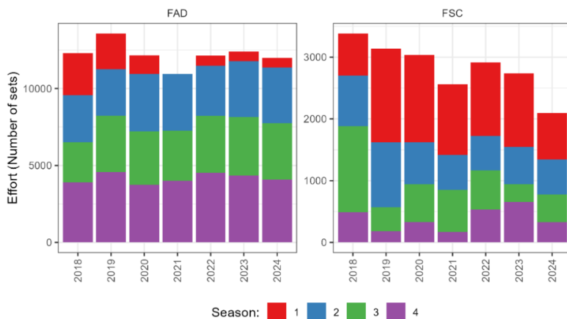
Figure 19.38.1. Tendances récentes de l'effort par saison de la pêcherie de senneurs opérant sur bancs libres (PSFS) et sous objets flottants (PSLS).
