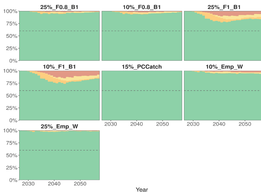
Figure 19.9.1. Série temporelle de l'état estimé du germon de l'Atlantique Nord selon les 7 CMP évaluées en 2026 dans le contexte du nouveau cadre de la MSE (ensemble de référence des modèles opérationnels). Pour chaque année, les couleurs indiquent la probabilité que le stock se situe dans chacun des quadrants de Kobe. La ligne pointillée indique que le stock a une probabilité de 60 % de se situer dans le quadrant vert du diagramme de Kobe.
