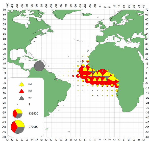
e. YFT (FAD/FREE 1991-2015)
