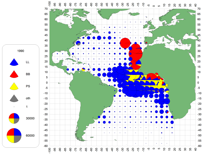
e. BET (1990-99)
