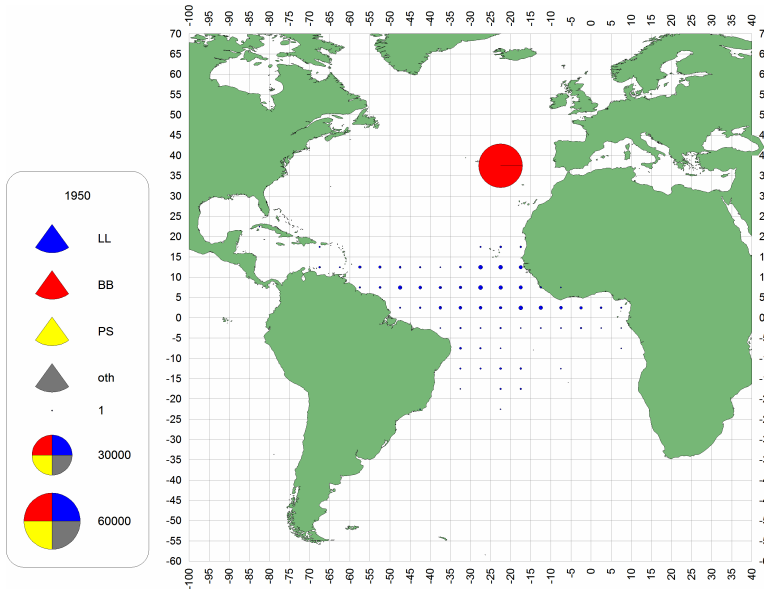
a. BET(1950-59)
