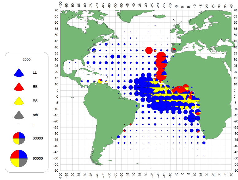
f. BET (2000-09)
