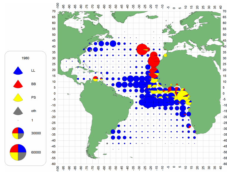
d. BET(1980-89)
