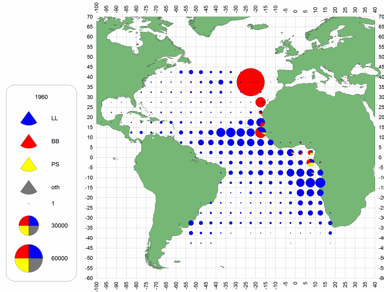
b. BET(1960-69)
