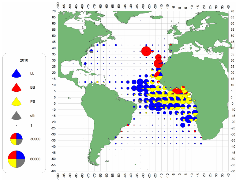
g. BET (2010-15)
