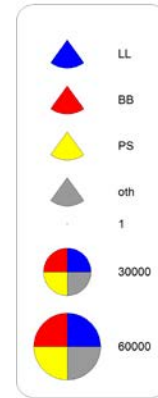
f. BET (2000-09)
