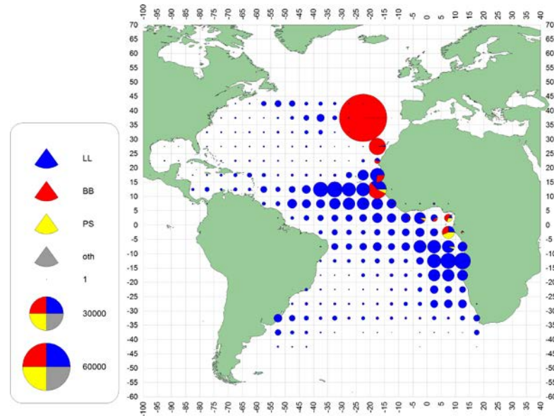
b. BET(1960-69)
