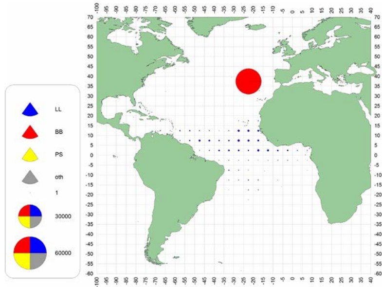
a. BET(1950-59)
