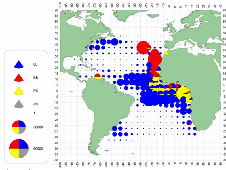
d. BET(1980-89)
