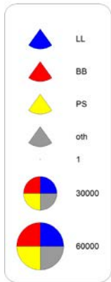
g. BET (2010-14)
