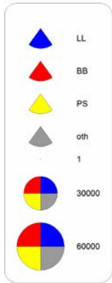
e. BET (1990-99)
