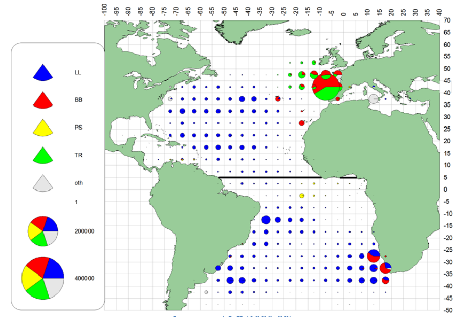
d. ALB(1980-89)
