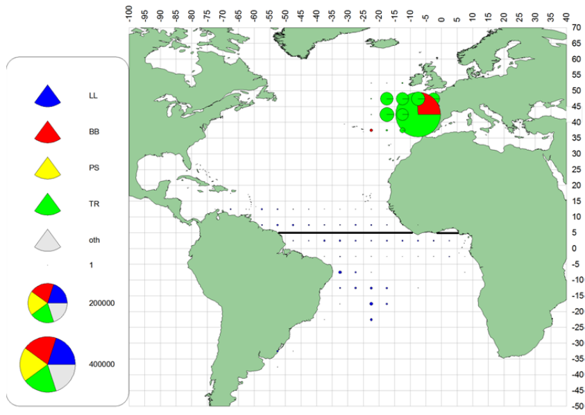
a. ALB(1950-59)
