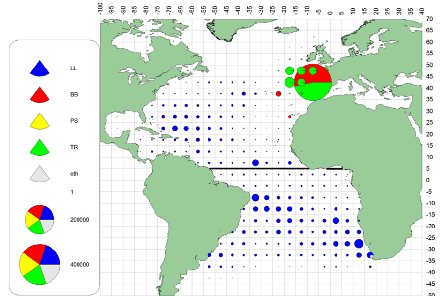
b. ALB(1960-69)
