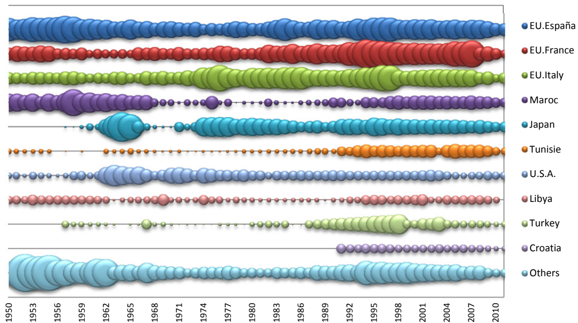
Figure 35 Relative BFT catch distribution by major Fleets. Ranking of catches based on the average amount of the five previous years. Figure 35 Distribution relative de la prise de BFT par flottille principale. Classification des captures sur la base de la moyenne des cinq dernières années. Figura 35 Distribución relativa de la captura de BFT por flotas principales. Clasificación de capturas en base a la media de los cinco últimos años.
