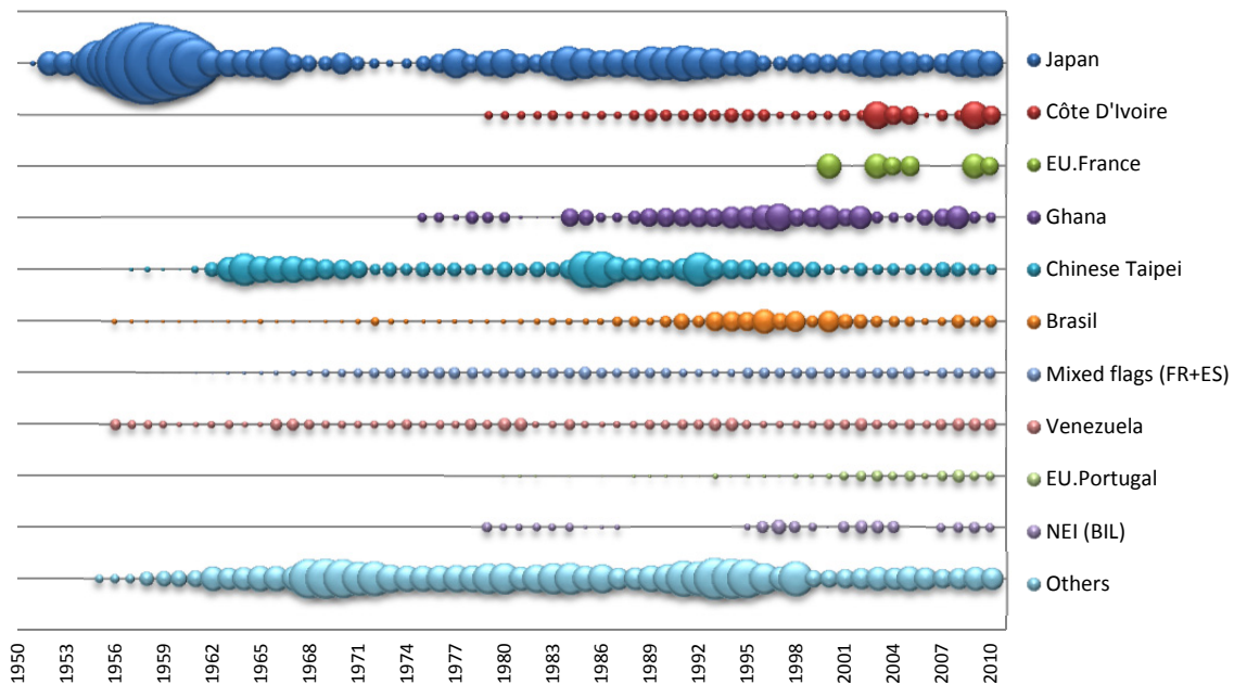
Figure 36 Relative BUM catch distribution by major Fleets. Ranking of catches based on the average amount of the five previous years. Figure 36 Distribution relative de la prise de BUM par flottille principale. Classification des captures sur la base de la moyenne des cinq dernières années. Figura 36 Distribución relativa de la captura de BUM por flotas principales. Clasificación de capturas en base a la media de los cinco últimos años.
