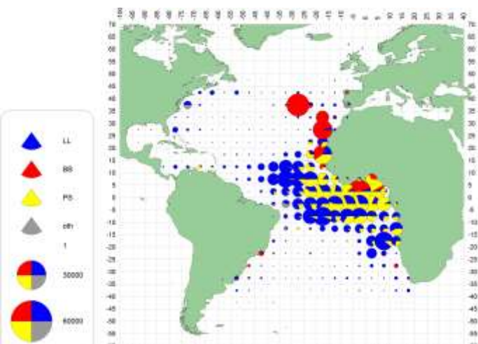
f. BET(2010-14)
