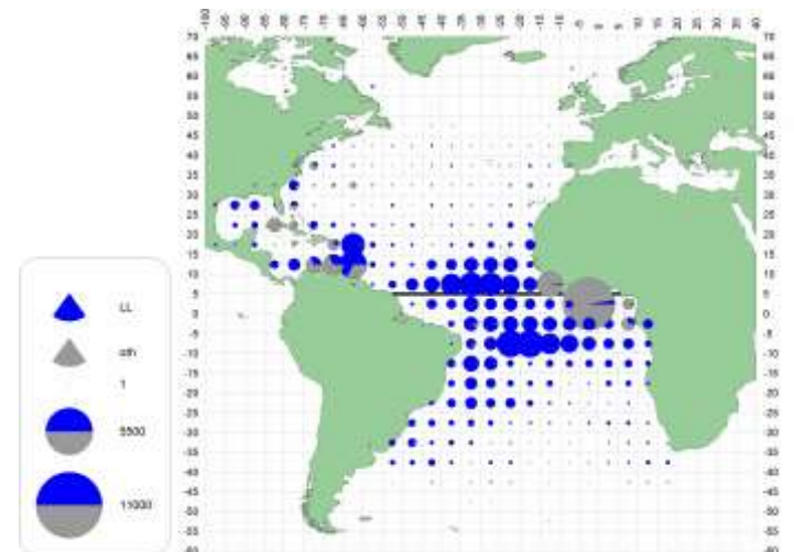
d. BUM (1990-99)
