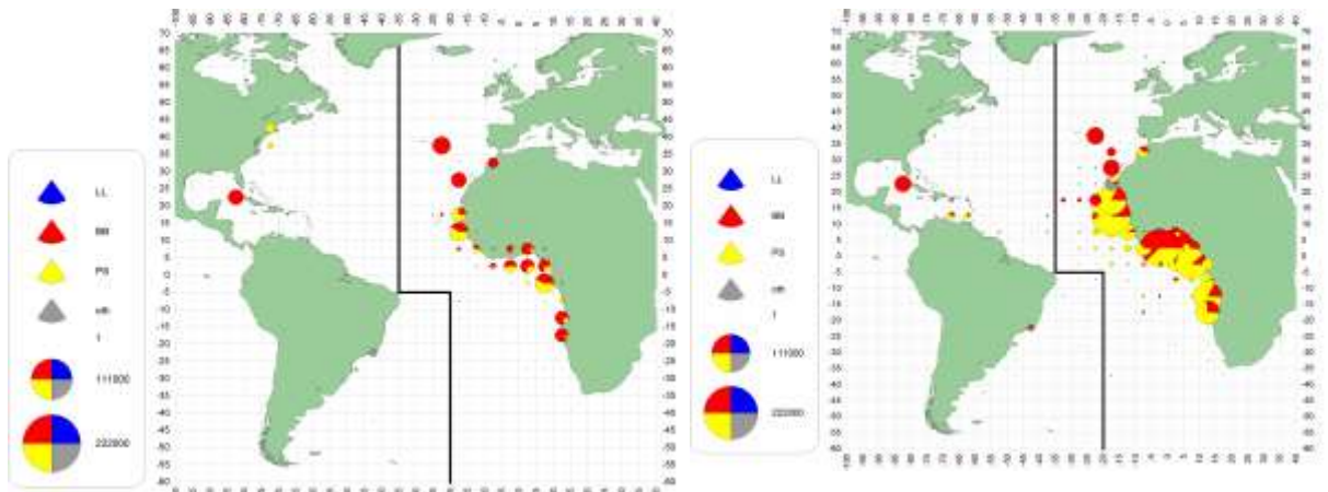
a. SKJ(1960-69)
