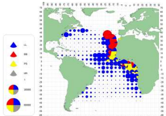
b. BET(1970-79)
