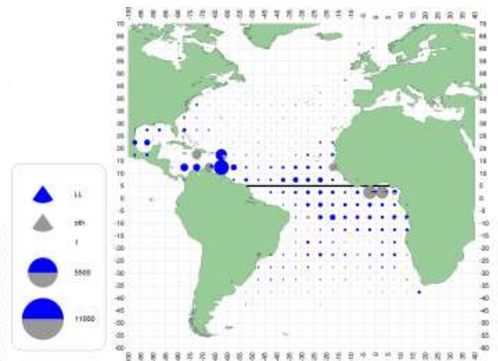
f. BUM (2010-14)
