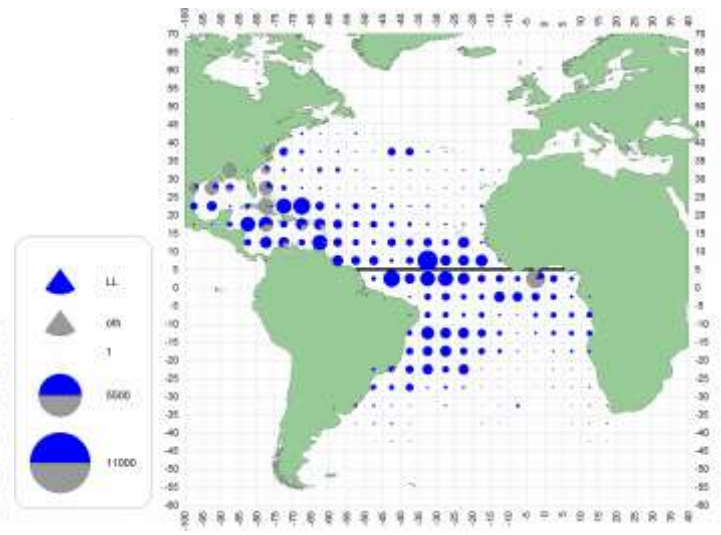
b. BUM (1970-79)
