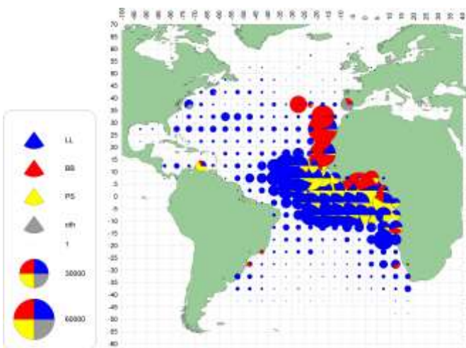
e. BET(2000-09)
