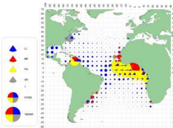
j. YFT (2000-09)
