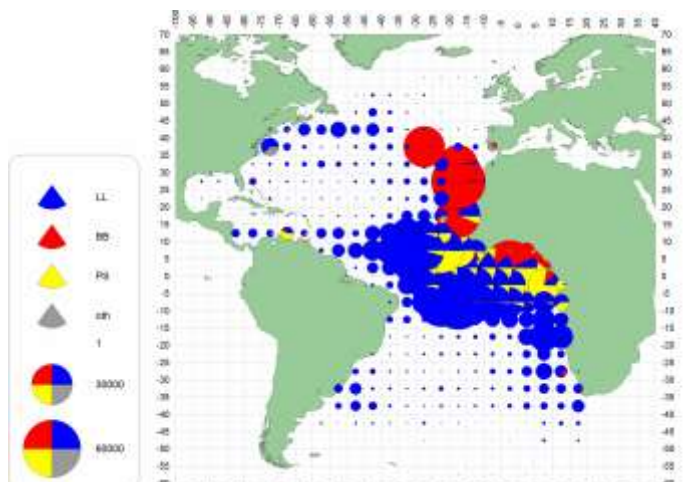
d. BET(1990-99)
