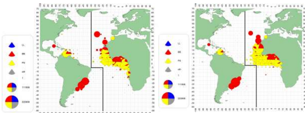
c. SKJ(1980-89)
