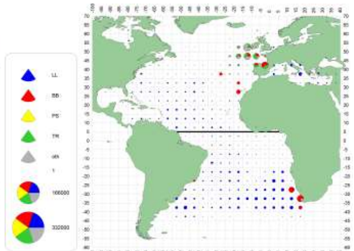
f. ALB(2010-14)
