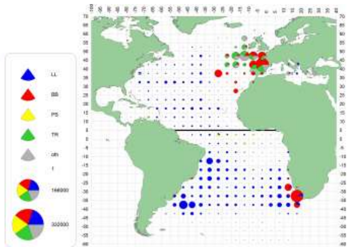
d. ALB(1990-99)
