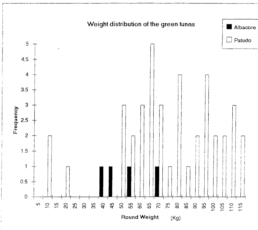
Figure 4: Distribution des poids individuels trois espèces de thons verts pêchés. On note la forte taille des patudos verts.
