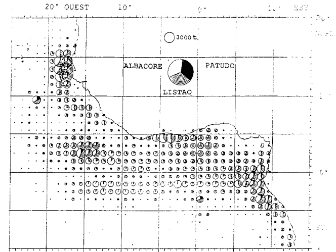
Prises toutes flottilles de surface, par espèce et carré de 1°, moyenne de la période 1980 à 1986. Catches of all surface fleets by species and 1° square, average of the period 1980 to 1986.
