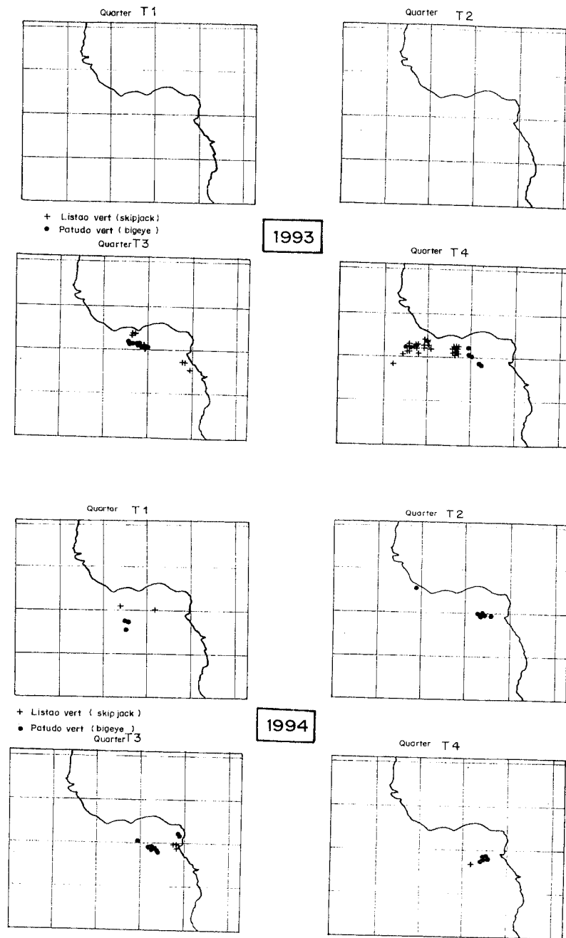
Figure 5 Cartographie trimestrielle des captures de listaos et patudos verts. A- 1993. Noter que les pêches de thons verts commencent au troisième trimestre. B- 1994
