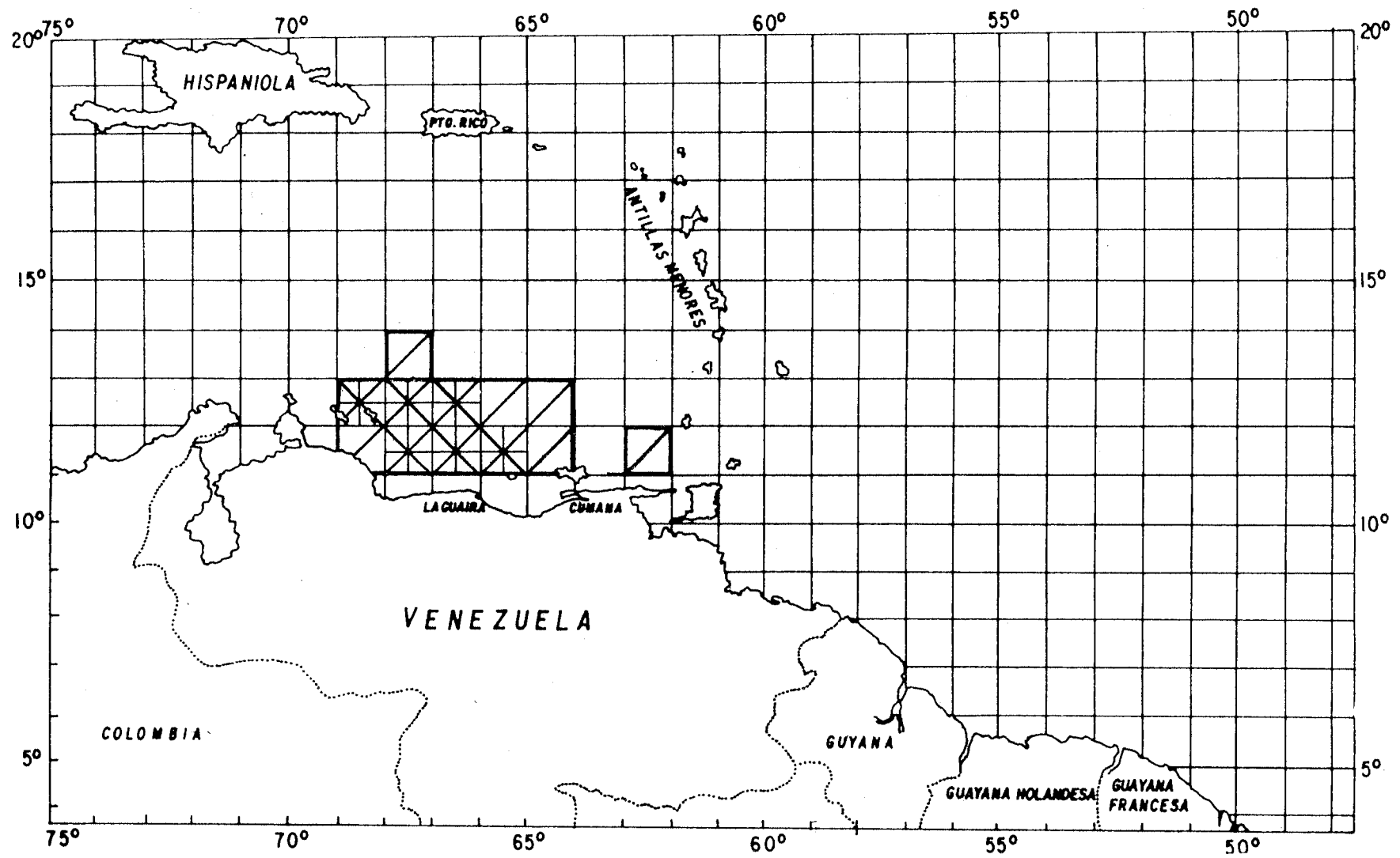
Fig. 1. Area general de procedencia y número de muestreos multispecíficos (▨). Se señalan las cuadrículas con mayor intensidad de muestreo (▩). Fig. 1. General area sampled and number of multispecies samples (▨). Squares with highest sampling intensity are shown (▩).
