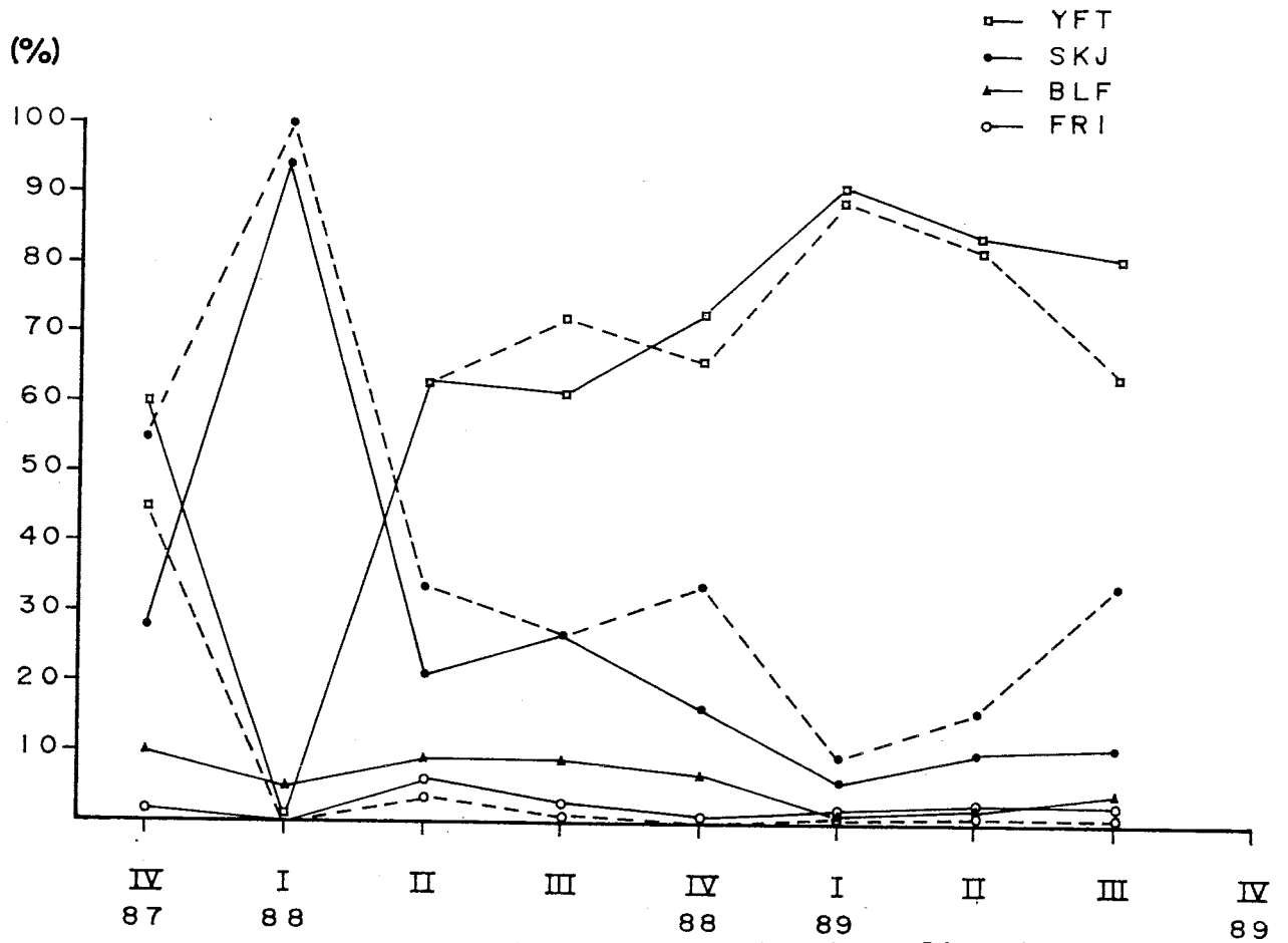
Fig. 2. Composición trimestral en porcentaje de las capturas venezolanas de superficie, según muestreos multispecíficos (—) y sus bitácoras correspondientes (-----), YFT (□), SKJ (•), BLF (▲), FRI (○).
