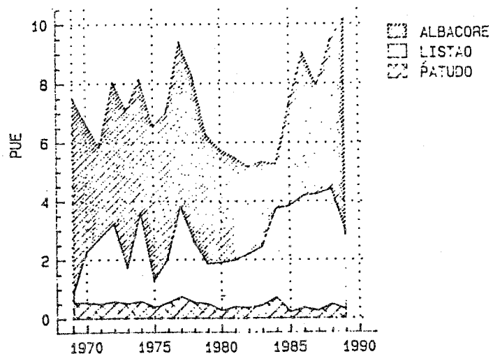
Figure 6.- PUE (t/jour) par espèces des grands senners FISM de 1969 à 1989.
