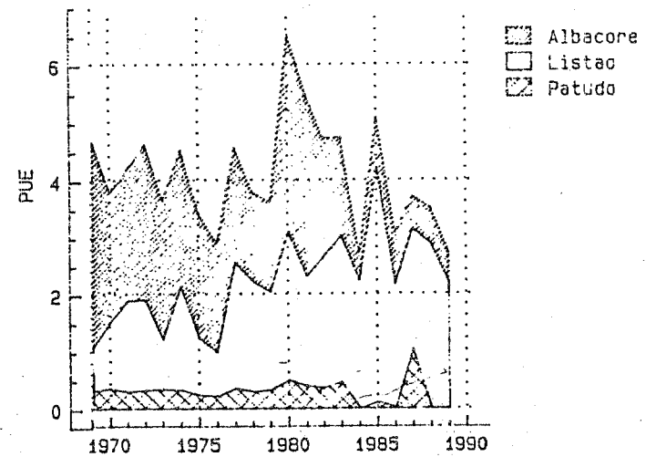
Figure 4.- PUE (tonne/jour par espèce des senneurs moyens FISM de 1969 à 1989.
