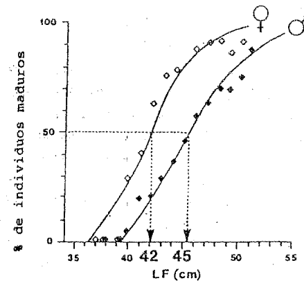
Figura 5.- Tallas de primera madurez de listado. (De Cayrè & Farrugio, 1986).
