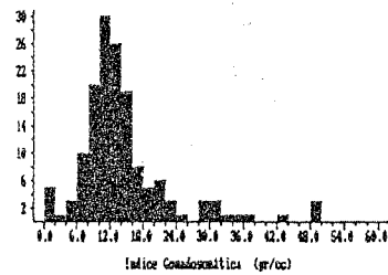
Figura 2.- Distribuciones de IGS de listado.
