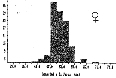
Figura 1.- Distribuciones de LF de listado en Canarias.
