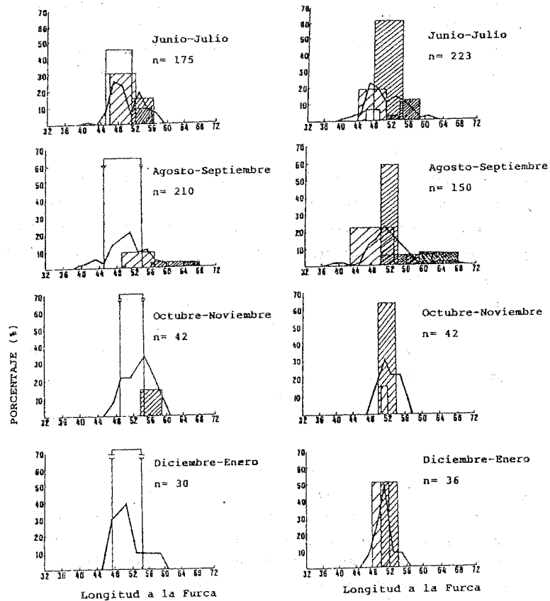
Figura 4.- Distribución de frecuencias de tallas de machos y hembras de listado en el área de Canarias y de Índices Gonadosomáticos para los mismos meses: (0-5) □, (5-10) ▨, (10-20) ▩, (20-30) ▤, (30-40) ▥, (>40) ▦.
