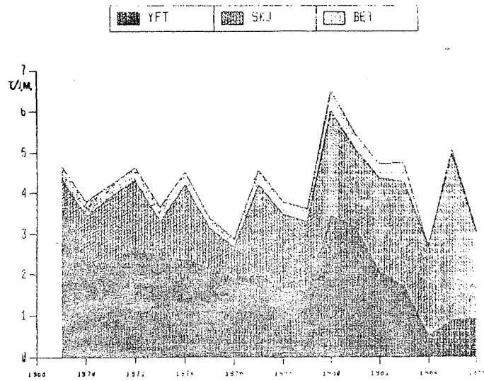
Figure 8. PUE par espèces des seneurs moyens FISM de 1969 à 1986
