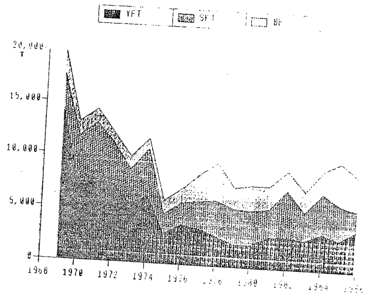
Figure 5. Prises par espèces des canneurs FIS de 1969 à 1986
