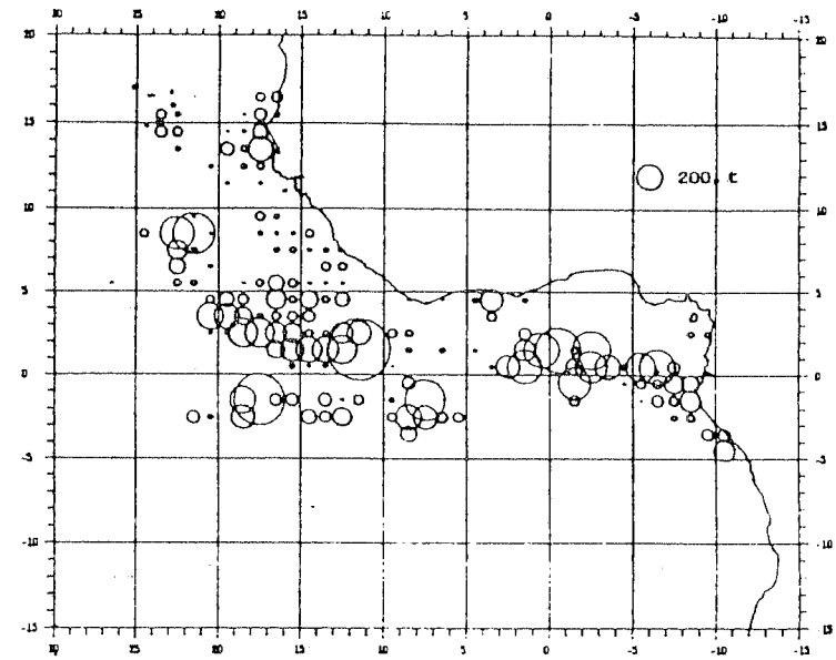
Figure 1. Prises d'albacore des senners FISM en 1982
