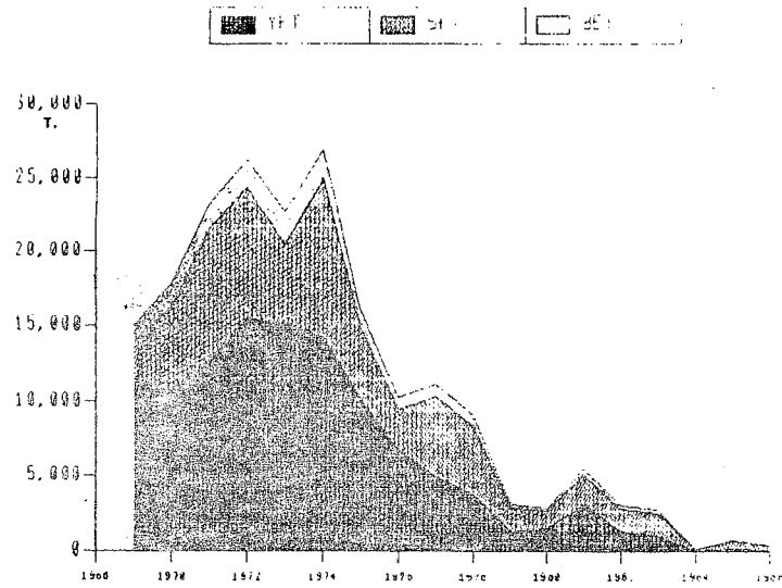
Figure 7. Prises par espèces des seneurs moyens FISM de 1969 à 1986
